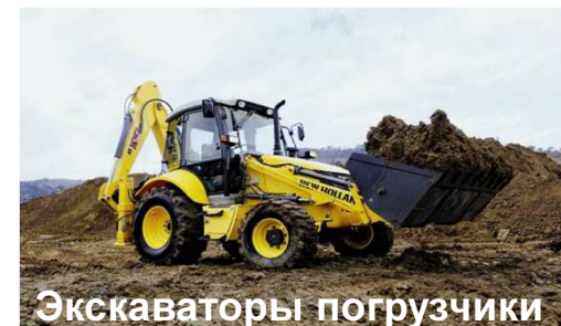
Экскаваторы
